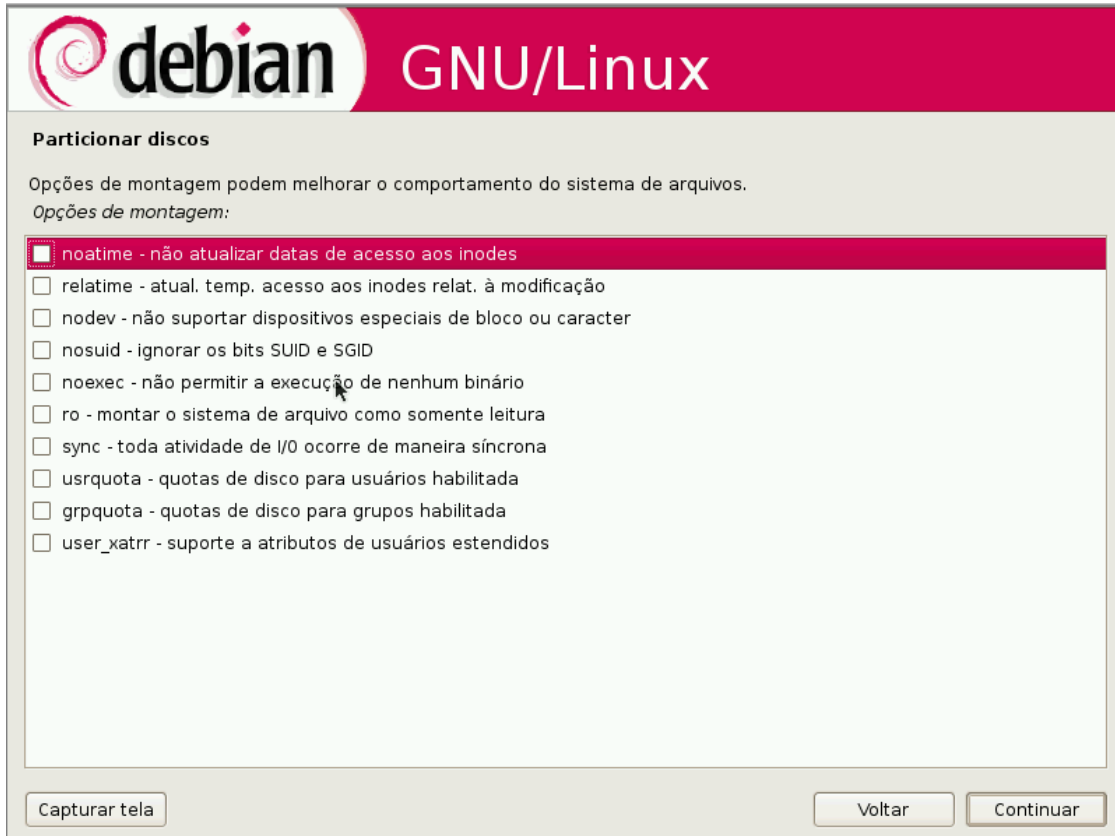
Ilustração 39: Opções do FSTAB
