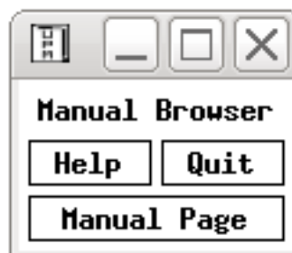
Ilustração 3: xman
