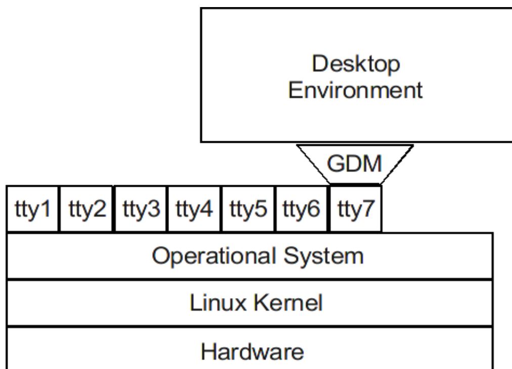
Ilustração 2: Estrutura do Sistema
