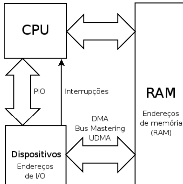
Ilustração 57: Arquitetura
