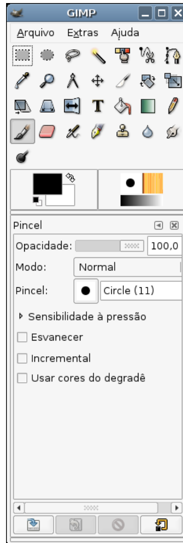
Ilustração 67: Gimp
