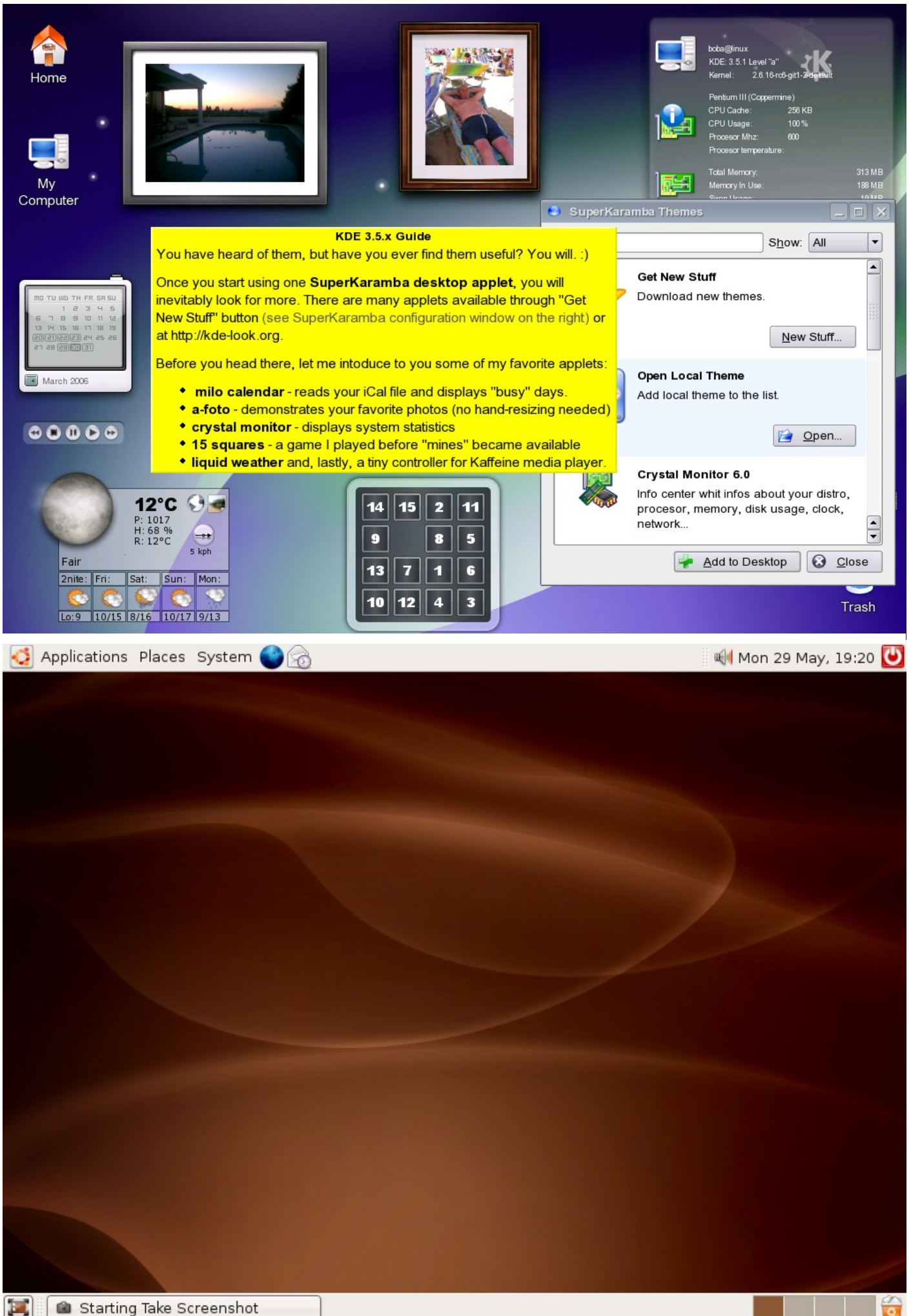
Ilustração 59: GNOME
